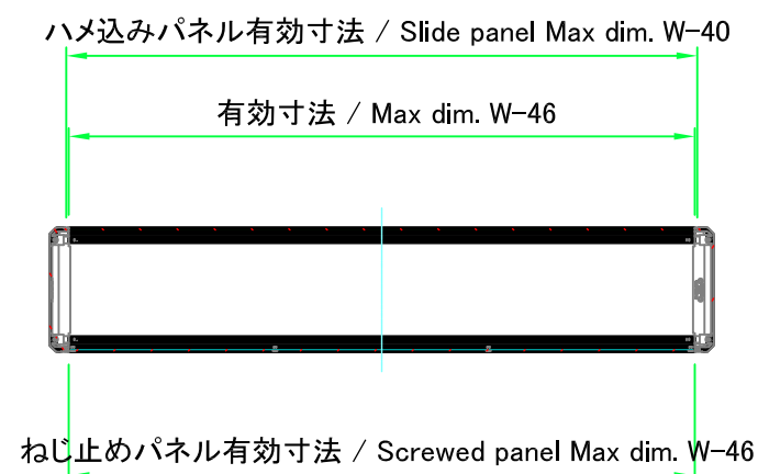
A-A ( 1 : 10 )
